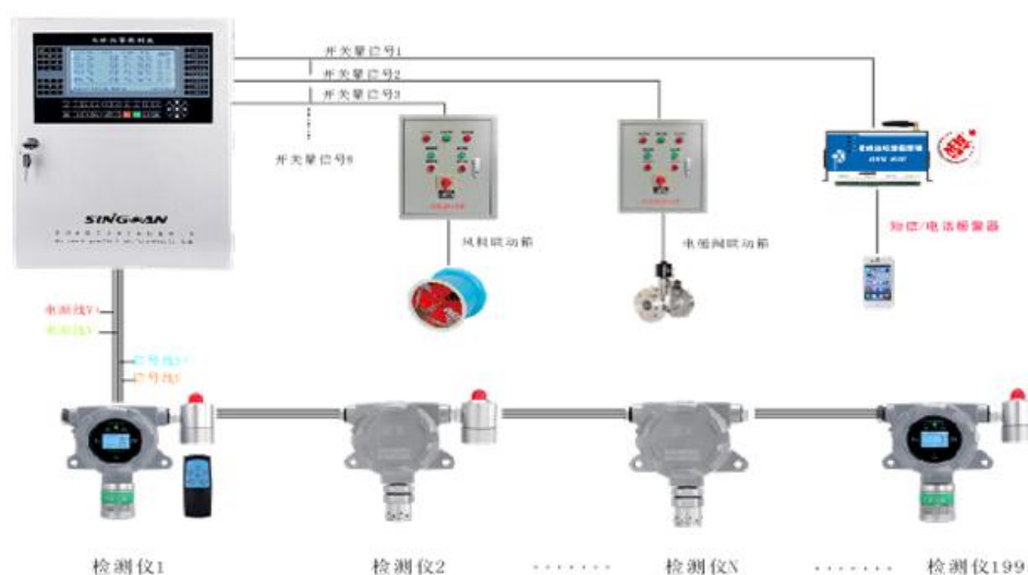
总线制示意图（液晶485通讯协议）
